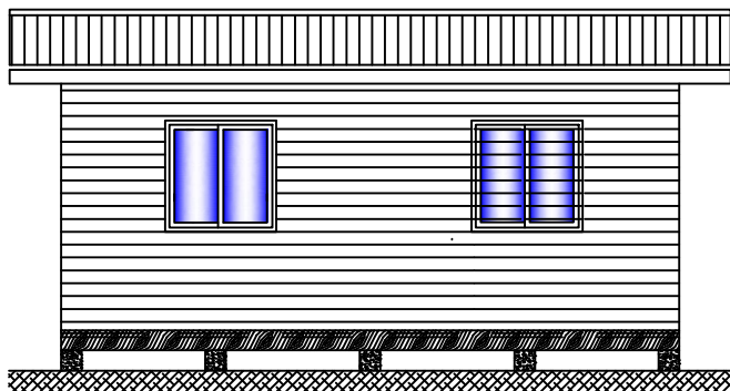
ELEVACION PRINCIPAL
