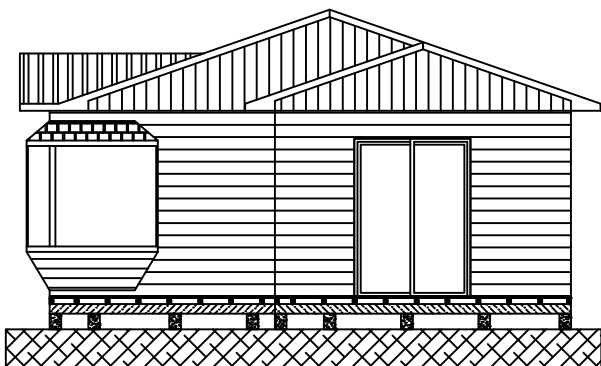
ELEVACIÓN LATERAL DERECHA Esc. 1/100
