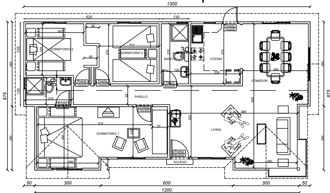
PLANTA DE ARQUITECTURA Esc. 1/50
