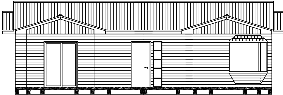
ELEVACION PRINCIPAL
