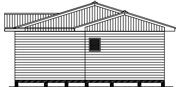
ELEVACION LATERAL IZQUIERDA
