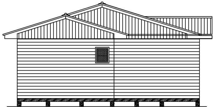
ELEVACION LATERAL IZQUIERDA ESC. 1:100
