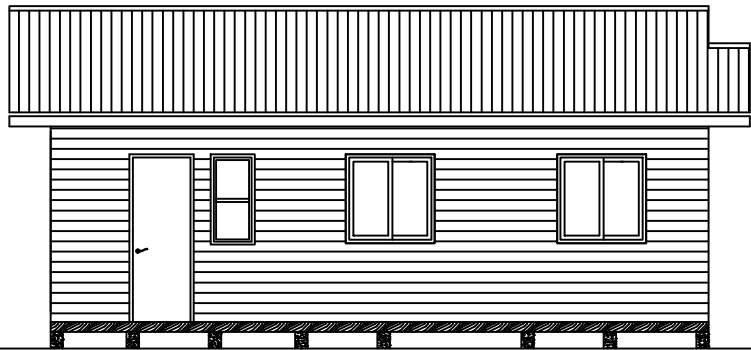
ELEVACION POSTERIOR ESC. 1:100
