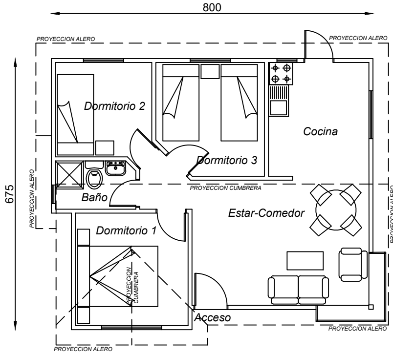
PLANTA DE ARQUITECTURA
