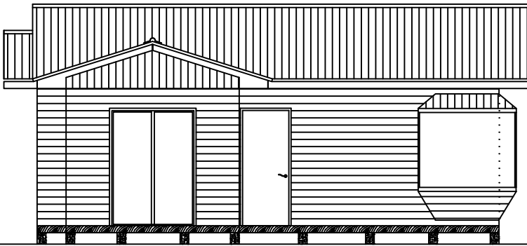
ELEVACION PRINCIPAL ESC. 1:100
