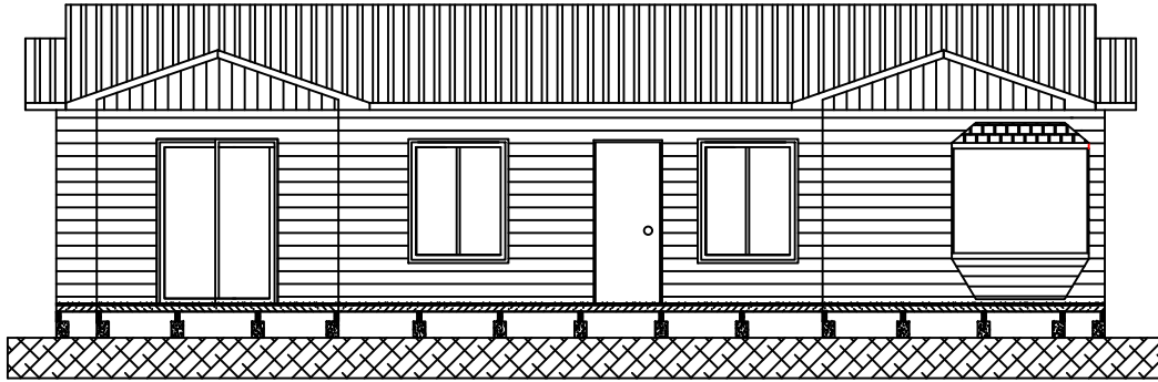
ELEVACIÓN PRINCIPAL
