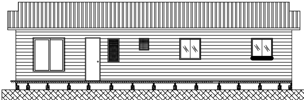
ELEVACIÓN POSTERIOR
