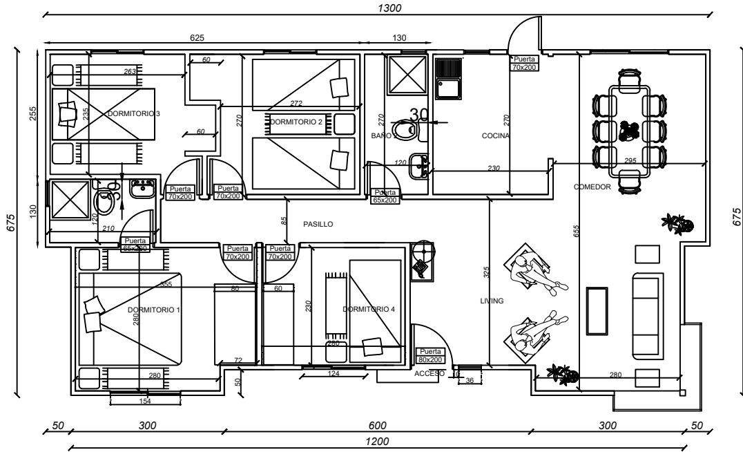
PLANTA DE ARQUITECTURA
