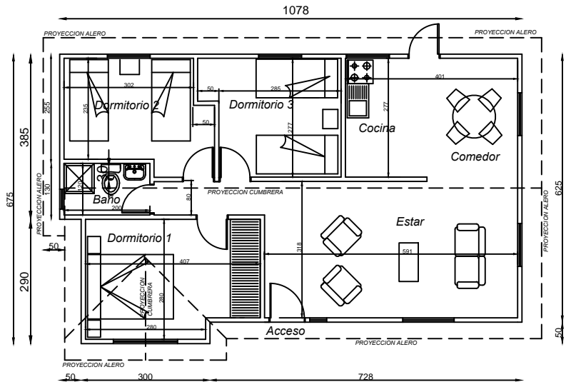
PLANTA DE ARQUITECTURA
