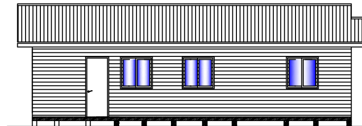
ELEVACION POSTERIOR ESC. 1:100
