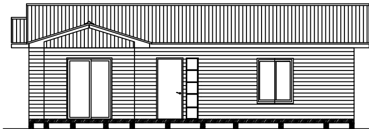
ELEVACION PRINCIPAL ESC. 1:100
