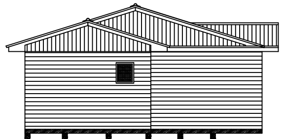
ELEVACION LATERAL IZQUIERDA
