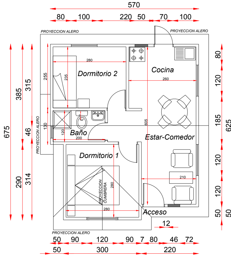
PLANTA DE ARQUITECTURA ESC. 1:100
