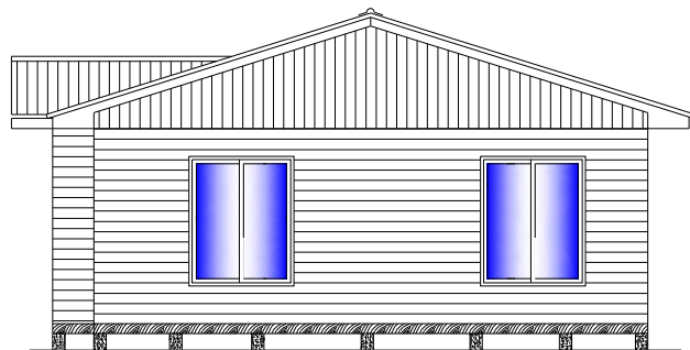
ELEVACION LATERAL DERECHA ESC. 1:100
