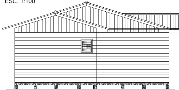
ELEVACION LATERAL IZQUIERDA ESC. 1:100
