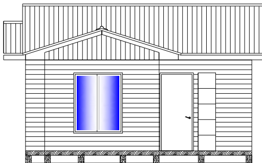
ELEVACION PRINCIPAL ESC. 1:100
