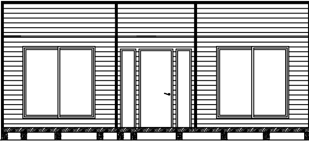
ELEVACION PRINCIPAL
