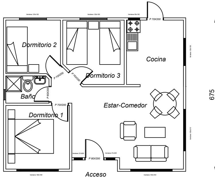
PLANTA DE ARQUITECTURA
