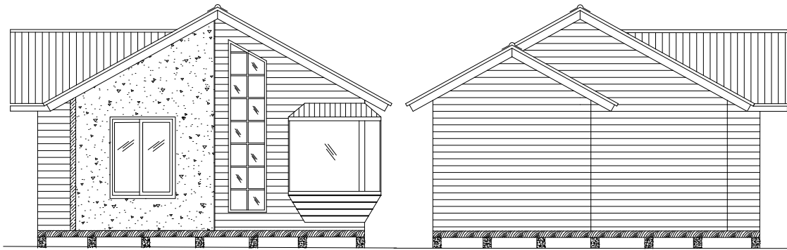
ELEVACION PRINCIPAL
